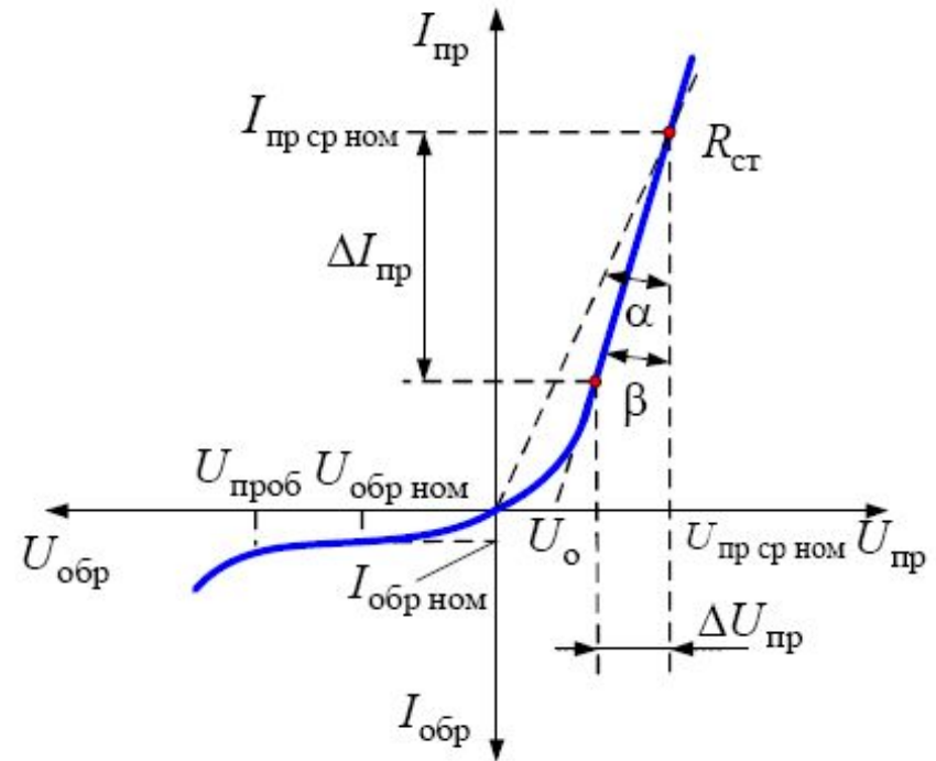
Рис 2.6. Вольт-амперная характеристика выпрямительного диода
