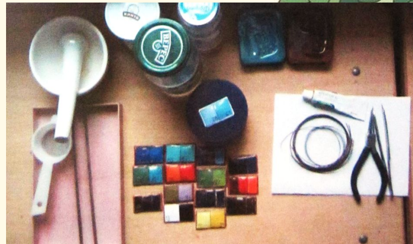
Сито, образцы эмалей, пинцеты, плоскогубцы, клей БФ-6, лоток для контрэмали
