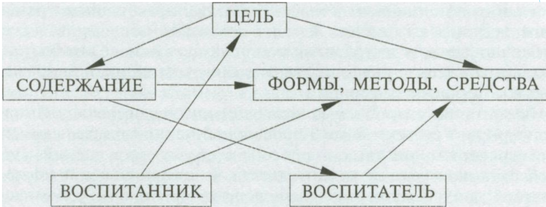
Рис. 1. Педагогическая система
