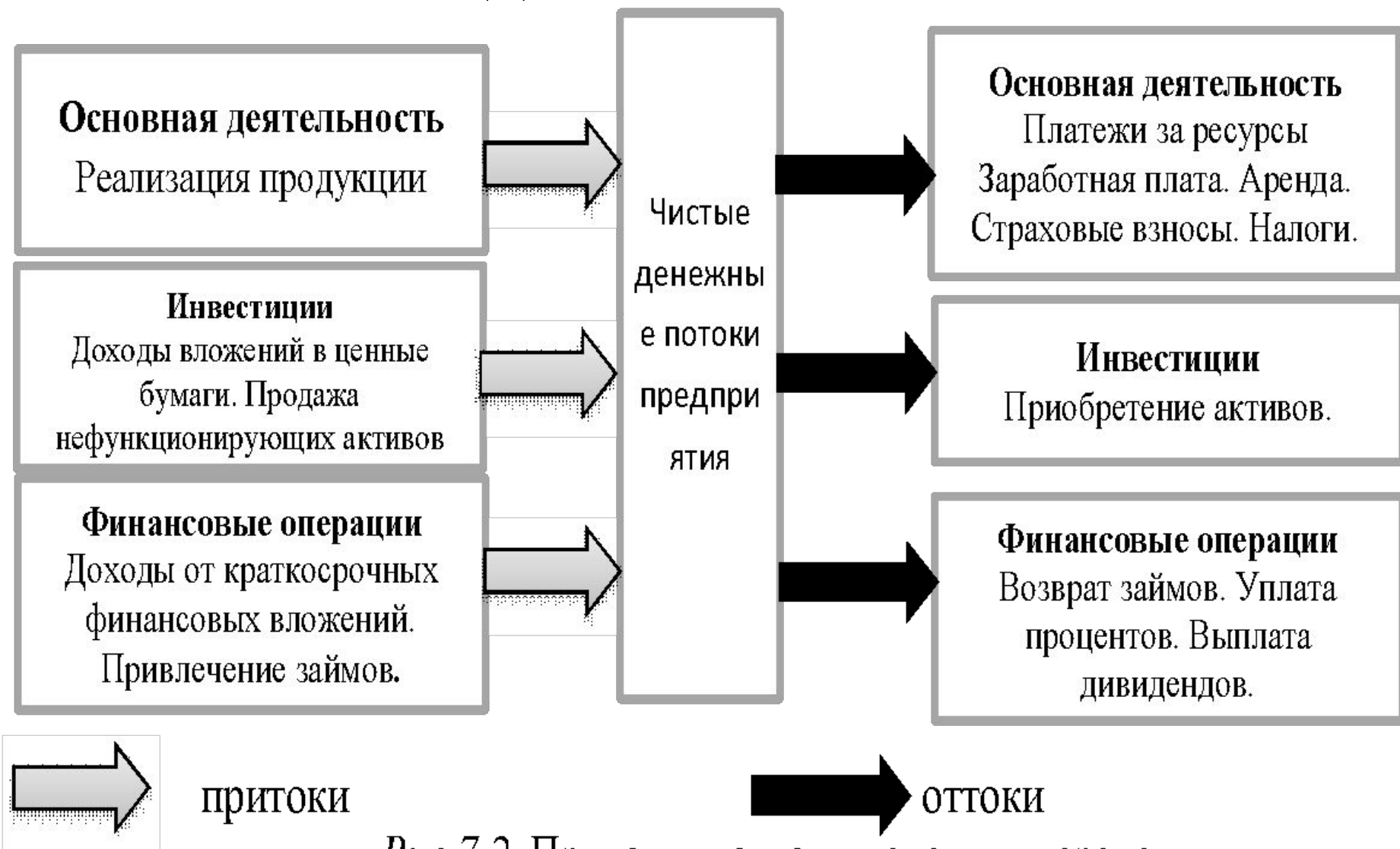
Рис. 7.2. Притоки и оттоки денежных средств.
