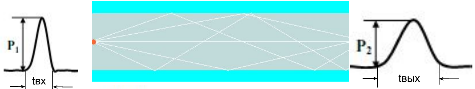
Выходной сигнал
