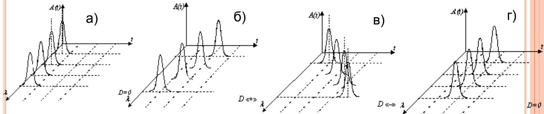
(а) импульс на входе; (б) нормальная дисперсия; (в) аномальная дисперсия; (г) область нулевой дисперсии
