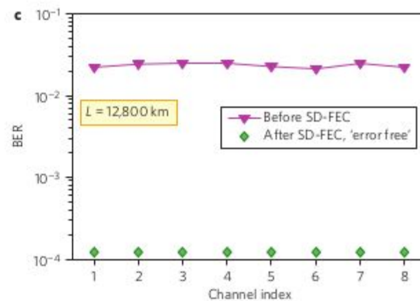
a. Схема экспериментальной установки. b. Сравнение качества сигнала с использованием новой схемы шумоподавления и без неё. c. Количество ошибок в сигнале, прошедшем 12800 км до и после коррекции ошибок
