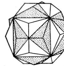
Пирит
