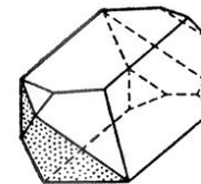
Ортоклаз
