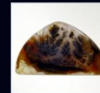
моховый
