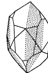
Бразильский
