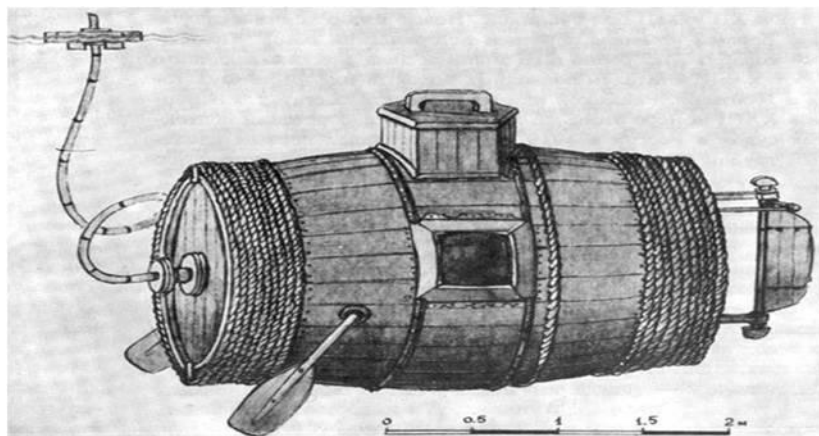
Подводная лодка Никонова
