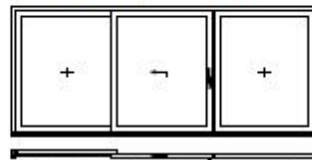
1 Hebe-Schiebeflügel, 2 Festverglasung
