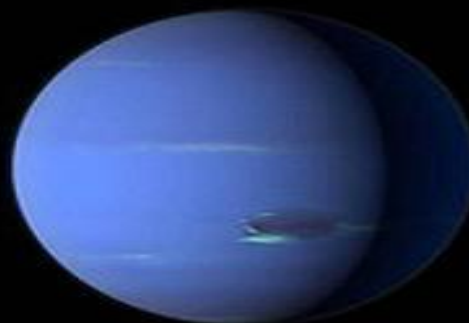
Нептун
