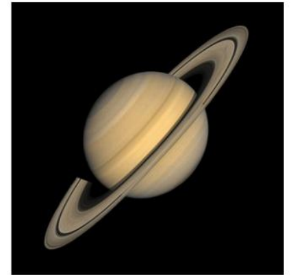
Сатурн
