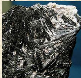
Эгирин
