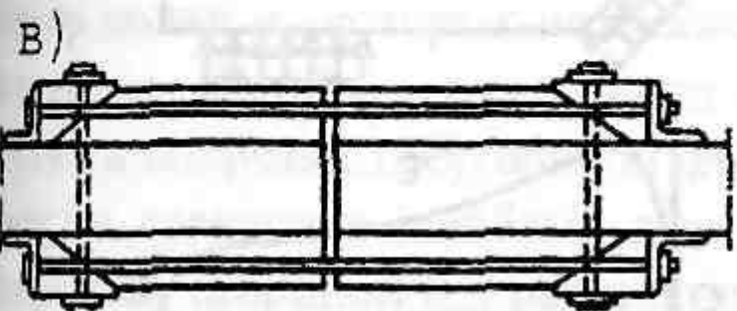
Стык с обжимными клиньями
