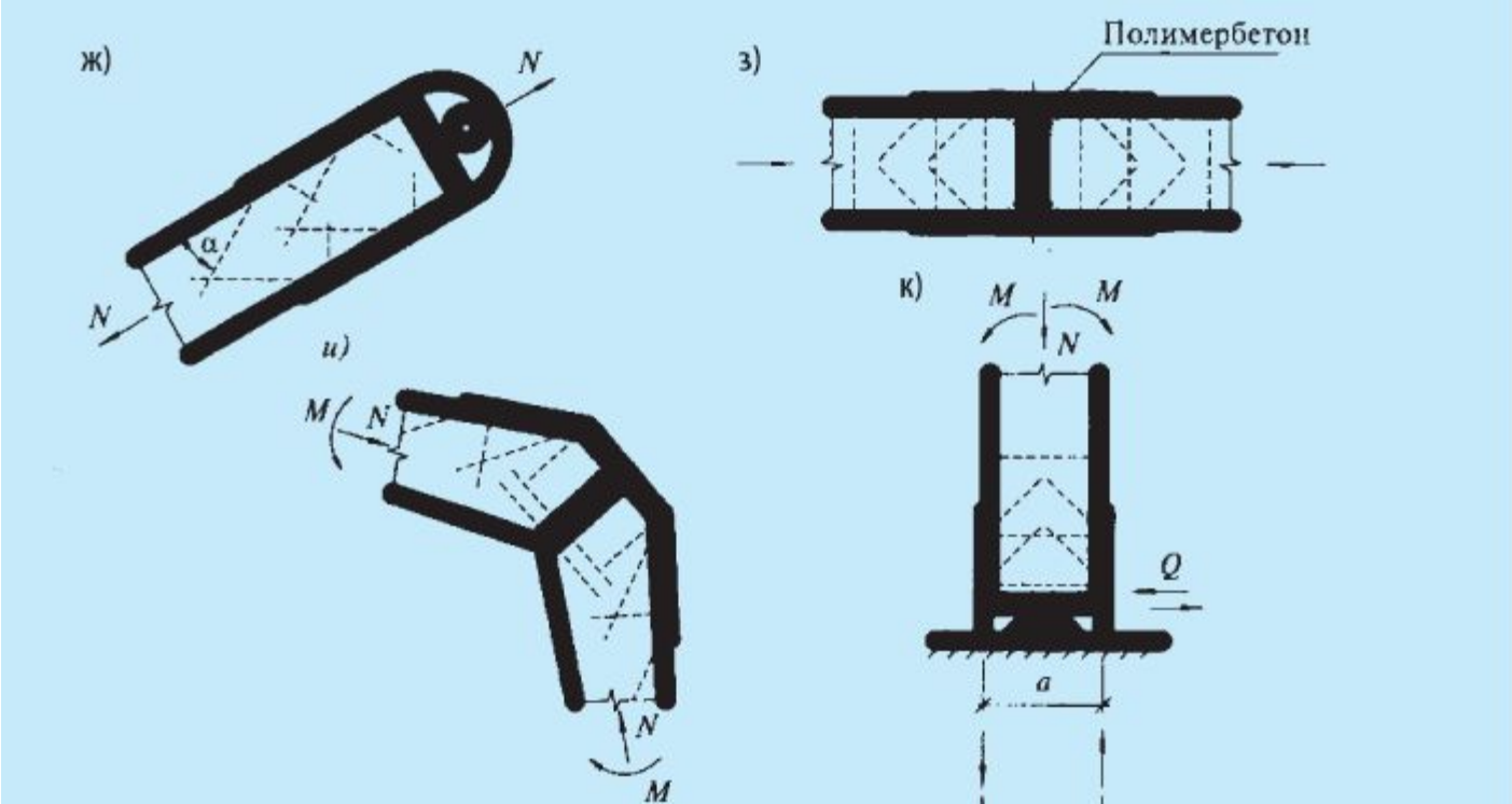
Рис.1. Используемые в проектировании соединения на наклонно вклееных стержнях [16]: а) — в виде связей составных элементов, б) — для повышения сдвиговой прочности клееной балки, в) — для анкеровки закладных деталей, г), д) — в опорных и других узлах конструкций; е) — схема симметричного универсального жесткого стыка элементов сечением <500 и >600; ж) — для растянутых элементов, з) — для сжатых стыков с полимербетоном, и) — для полигональных элементов, несимметричная схема (карниз рамы), к) — для узла защемления стоек.
