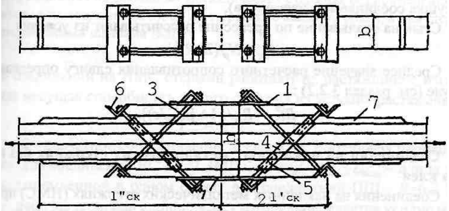
Стык с двойным обжимом
