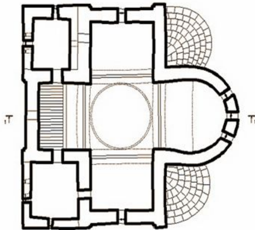
ПЛАН II ЯРУСА
