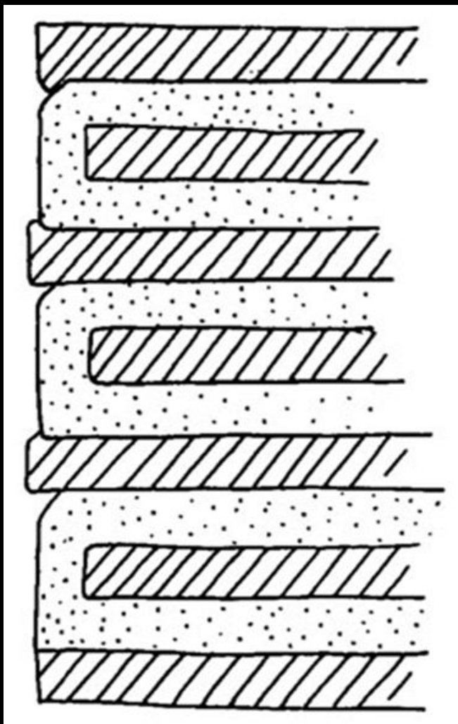
Киев. Софийский собор. Схема кладки с заглубленными рядами.
