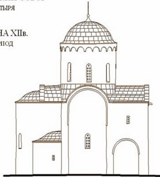
СЕВЕРНЫЙ ФАСАД
