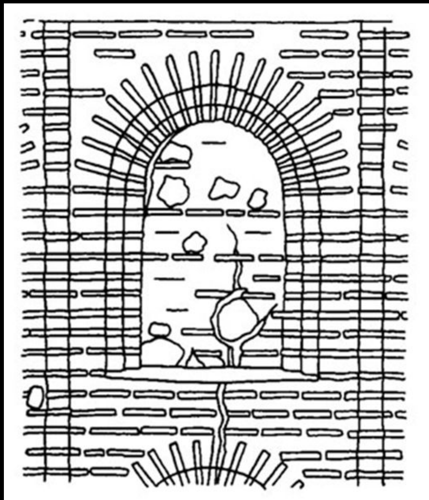
Киев. Софийский собор. Схема кладки с заглубленными рядами.
