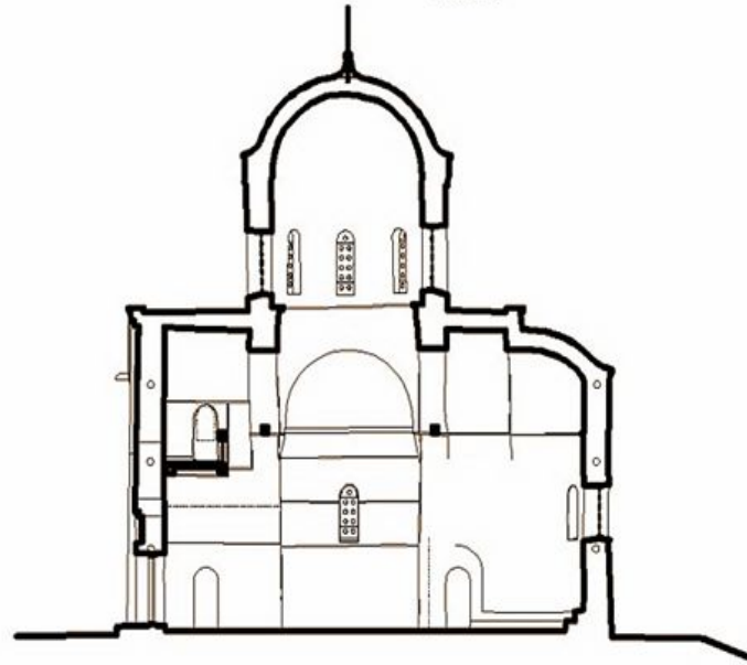
РАЗРЕЗ 1-1
