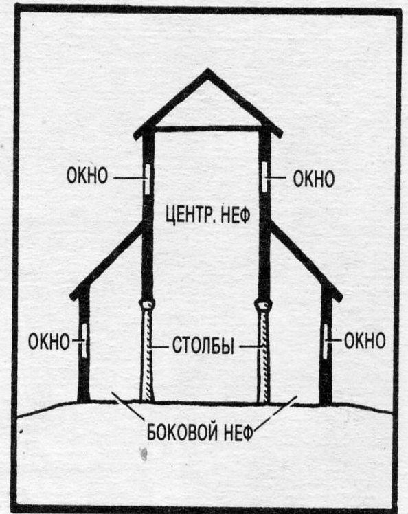
Разрез базилики.
