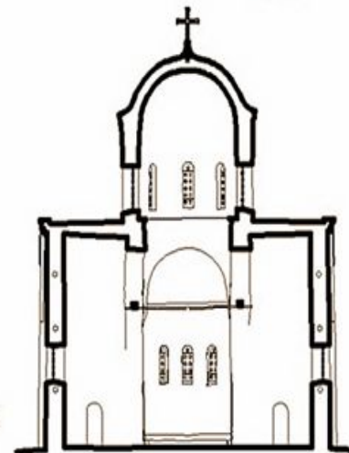
РАЗРЕЗ 1-1
