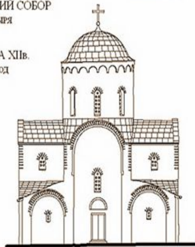
ЗАПАДНЫЙ ФАСАД
