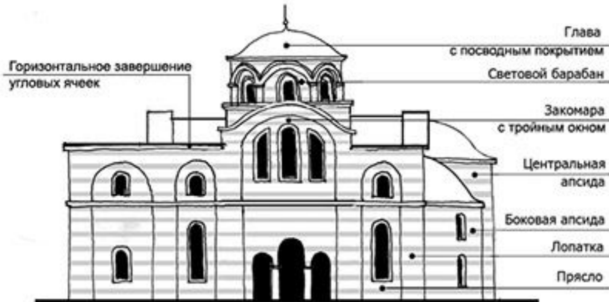
Фасад византийского храма
