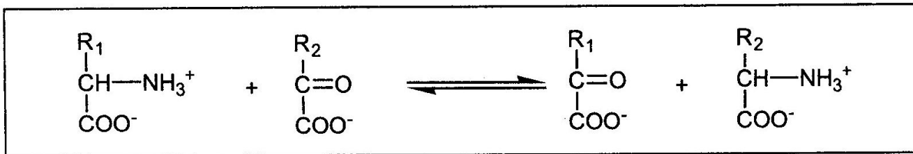
Рис. 20.5. Трансаминирование аминокислот.
