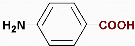
п-аминобензойная кислота
