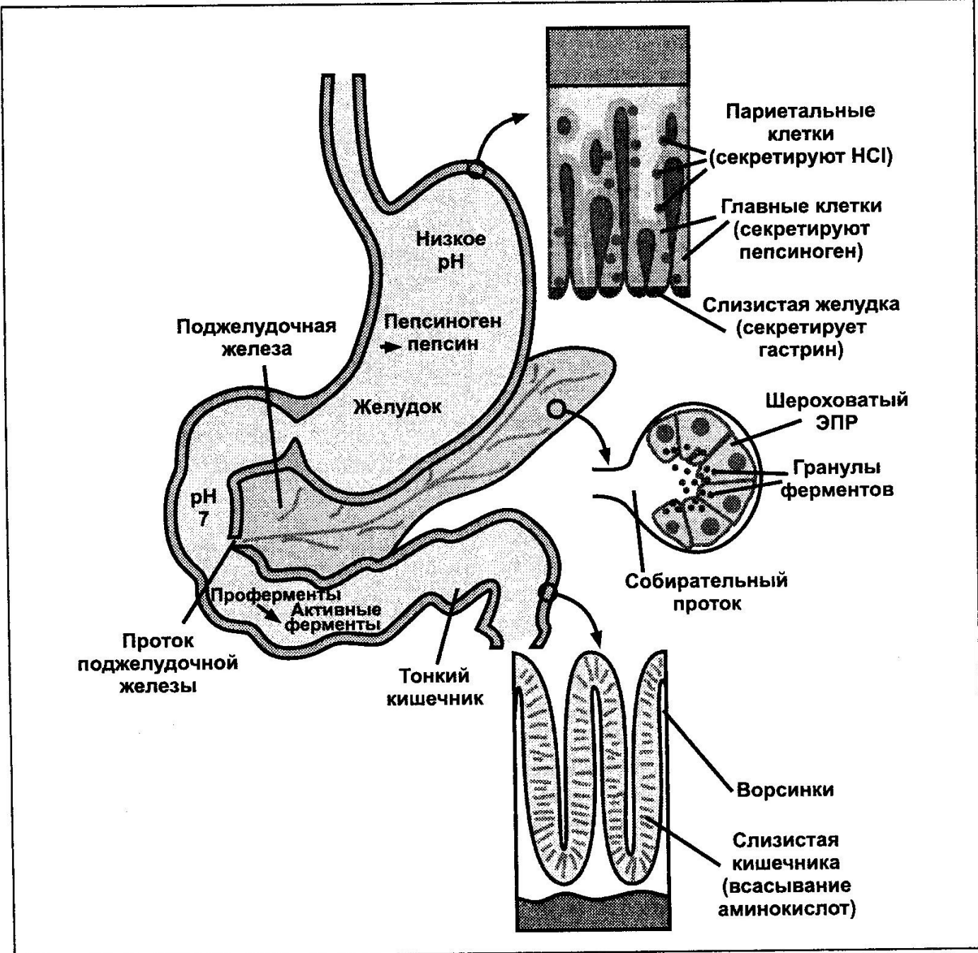
Рис. 20.1. Переваривание белков.
