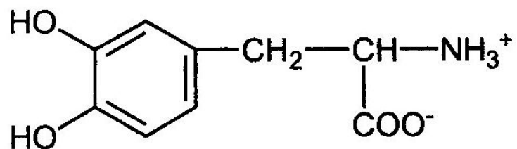
ДОФА
