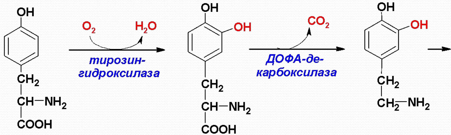
ДОФА
