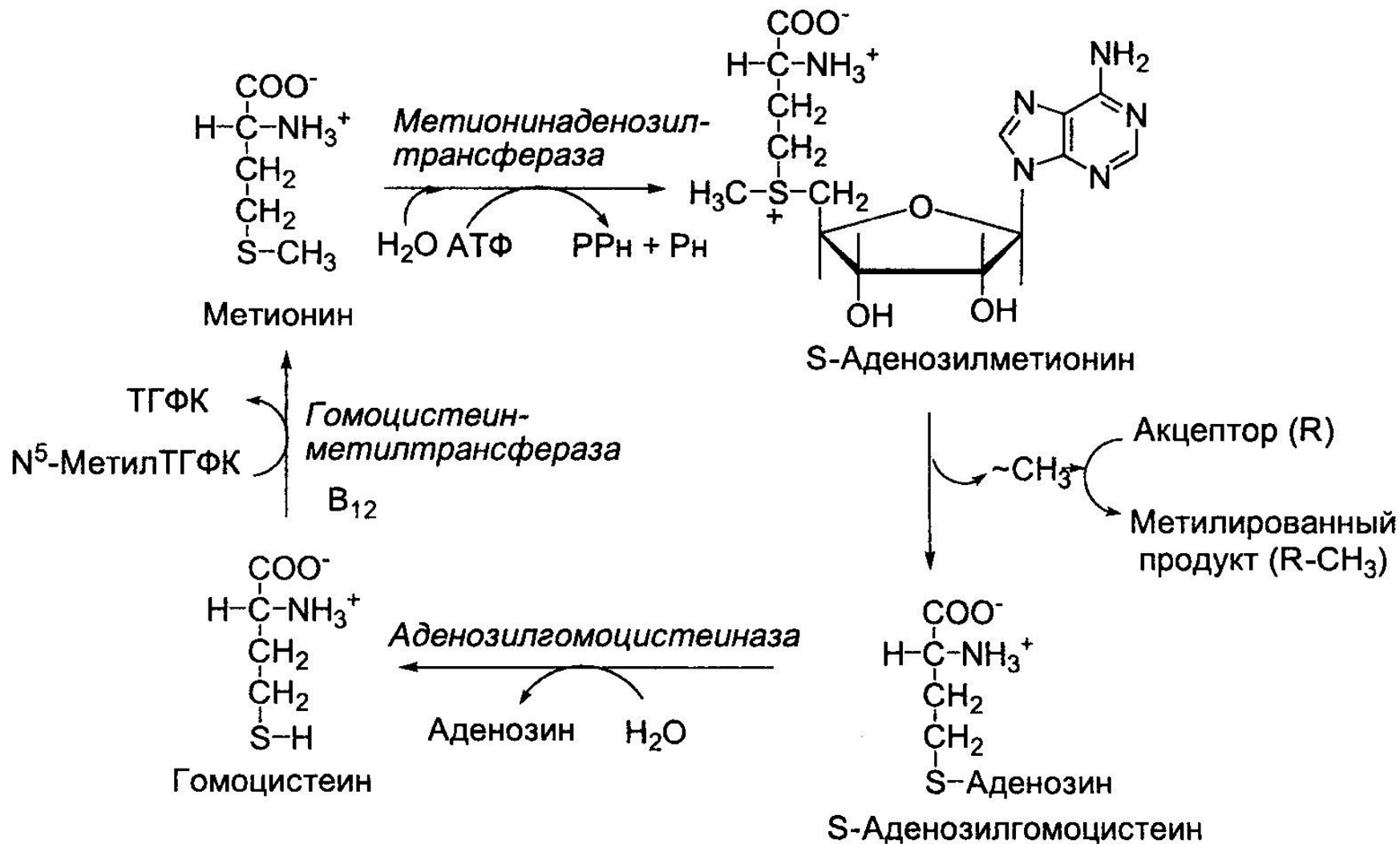
Рис. 22.2. Трансметилирование.
