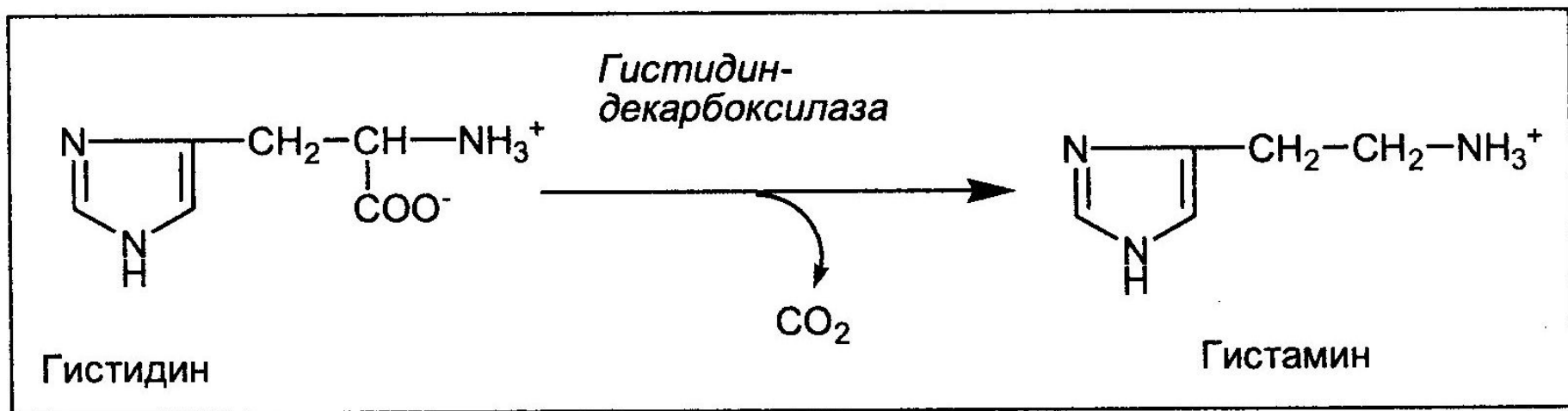
Рис. 20.14. Синтез гистамина.
