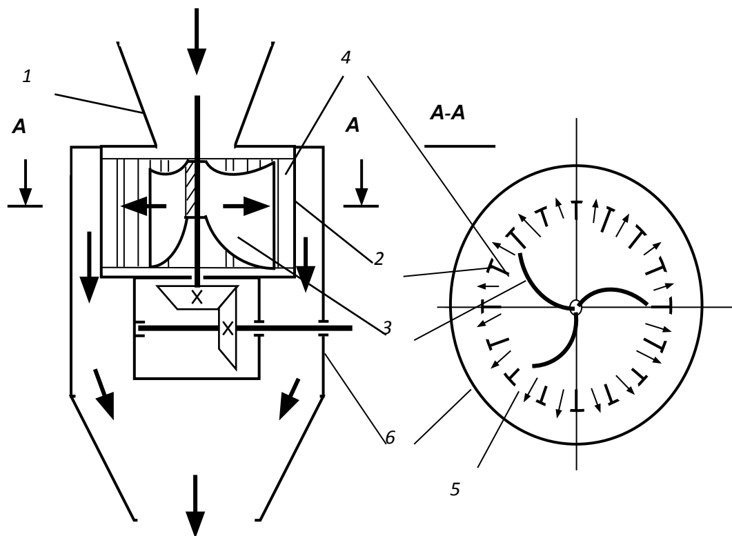
Схема и внешний вид центробежной свеклорезки
