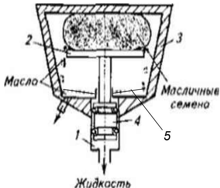
Схема гидравлического прессы.
