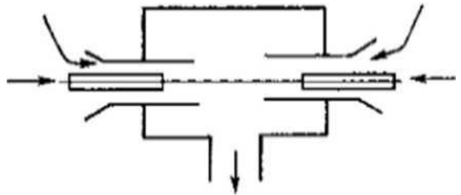
б) струйная мельница
