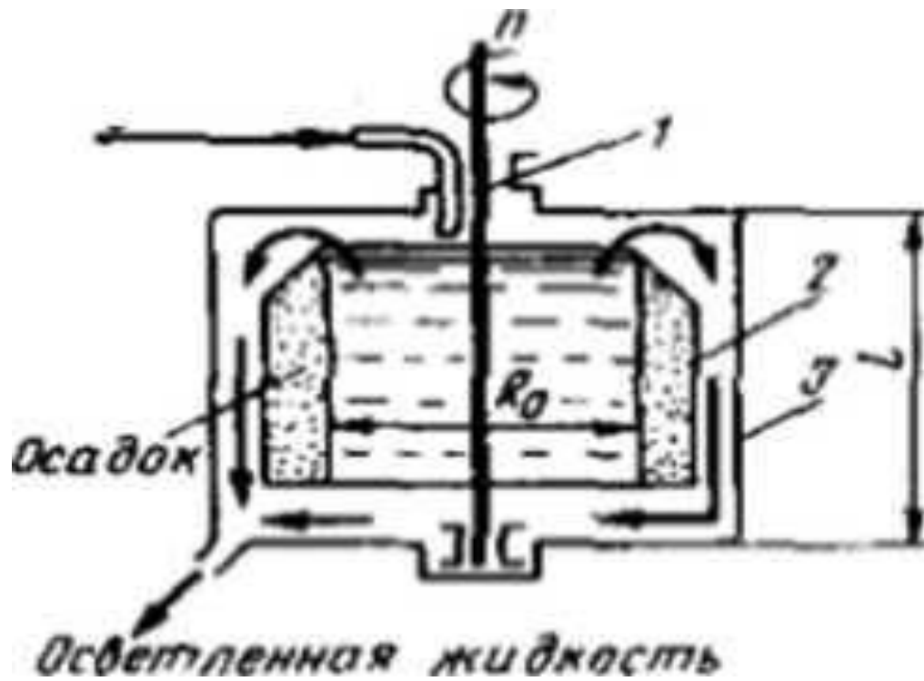
Рис 7. Отстойная центрифуга:
