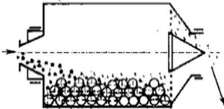
а) шаровая (стержневая) мельница
