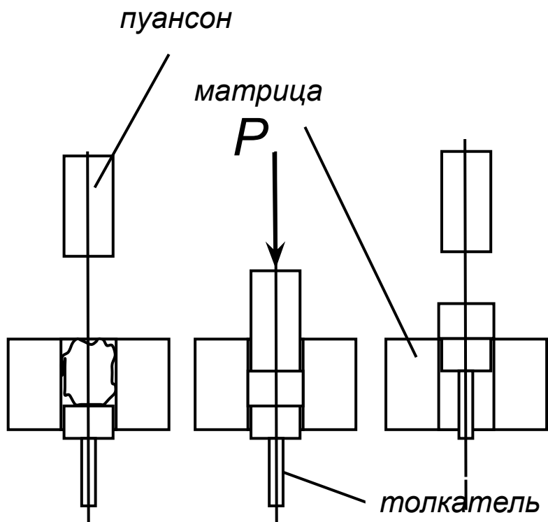
Схема штампования
