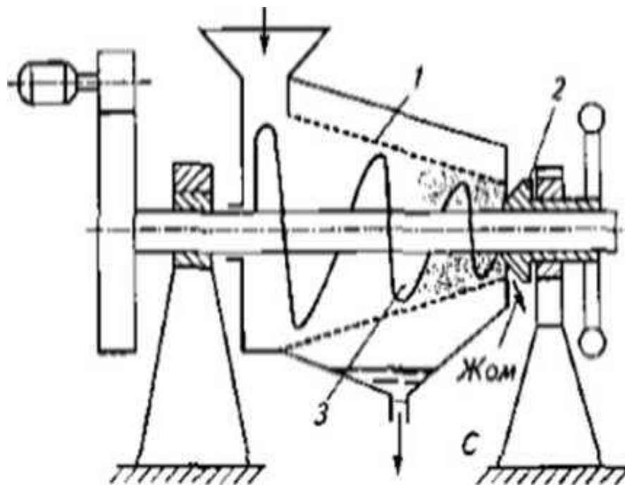
Схема шнекового зернового прессы
