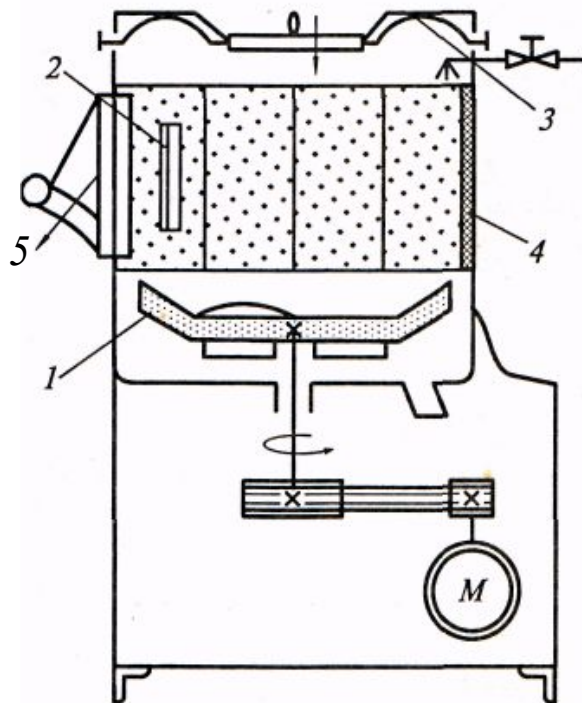
Схема картофелеочистительной машины :
