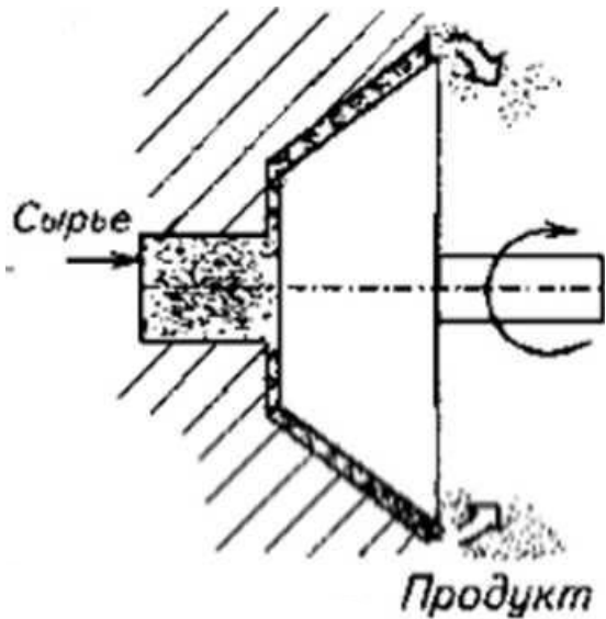
в) коллоидная мельница
