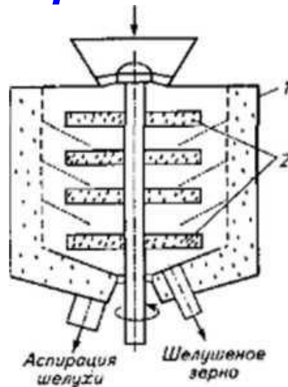
Схема зерношелушителя;
