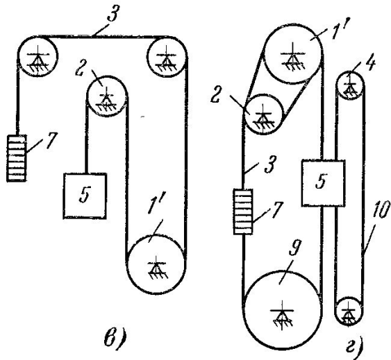
Кінематичні схеми ліфта
