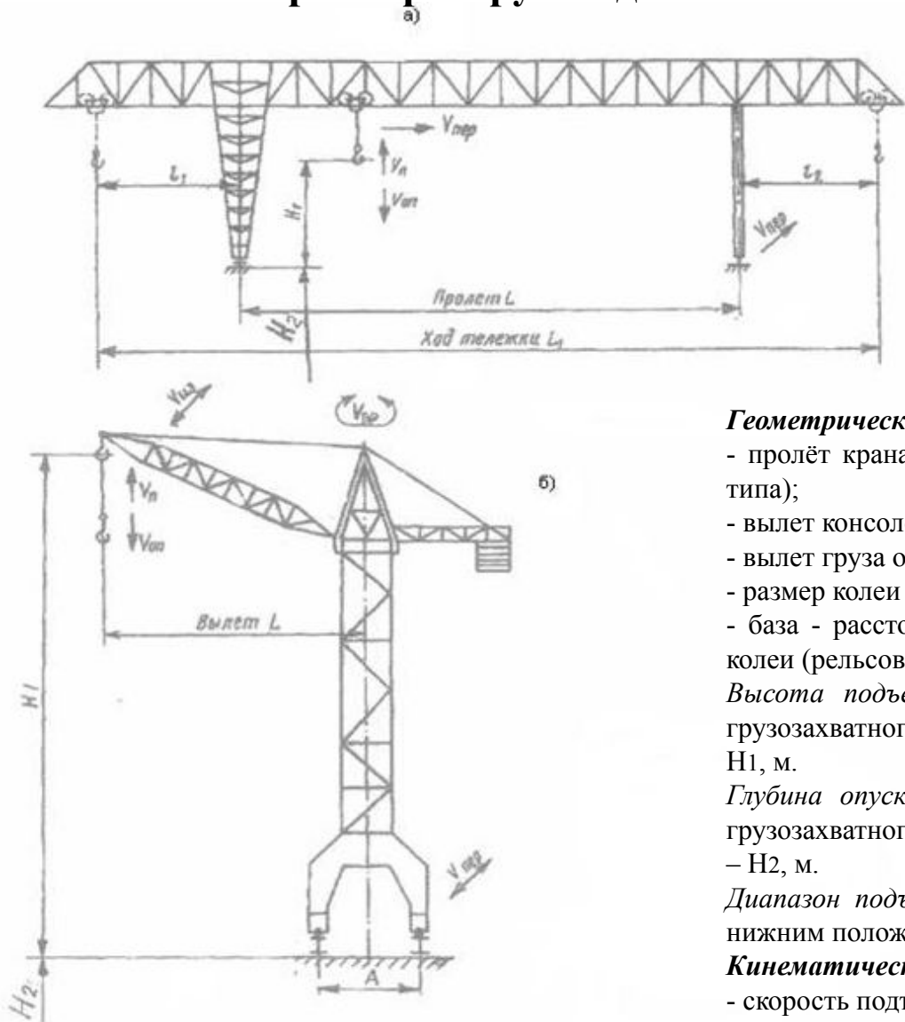
Рис. 2. основные геометрические и кинематические характеристики кранов:
