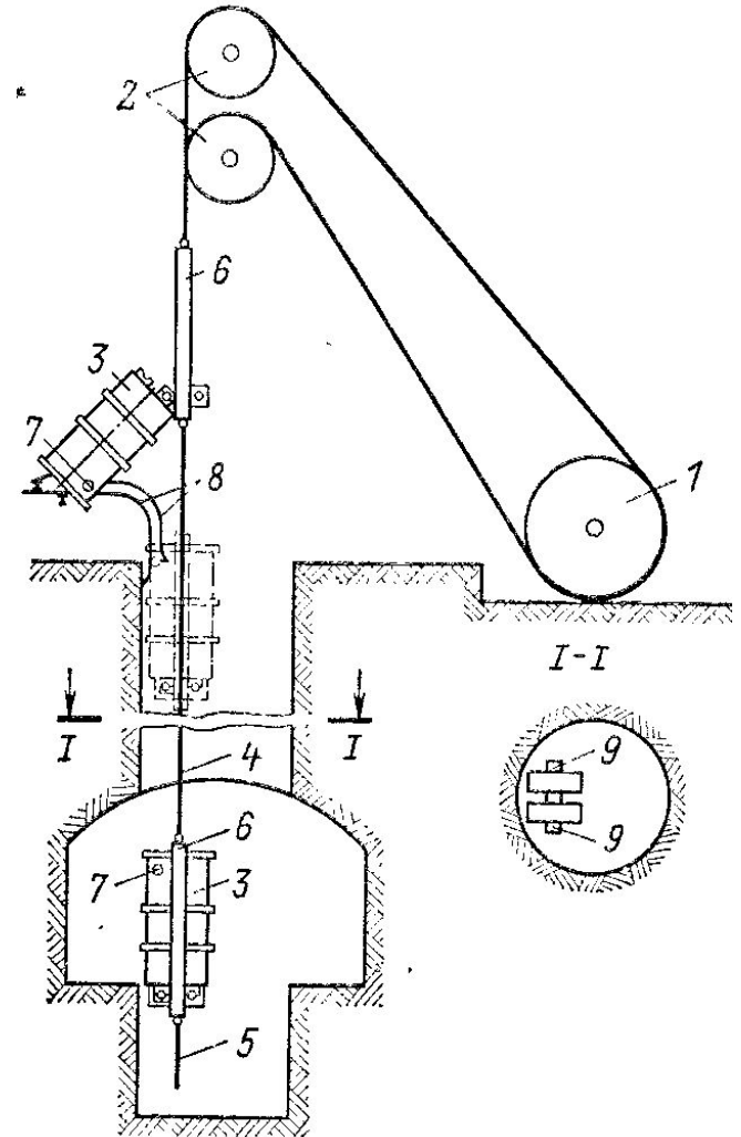
Кінематична схема шахтного підйомника:
