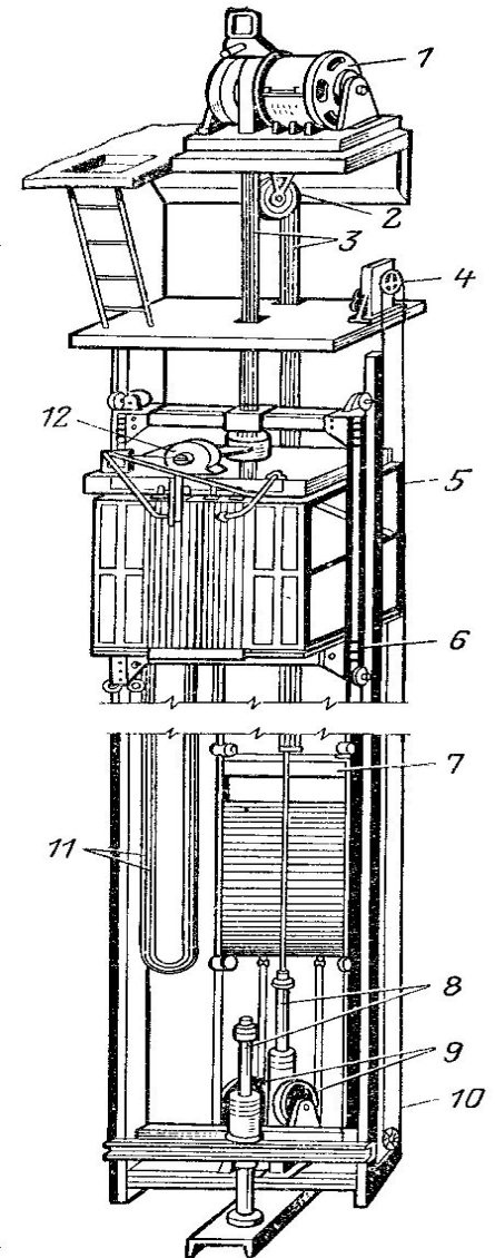
Загальний вигляд пасажирського швидкісного ліфта
