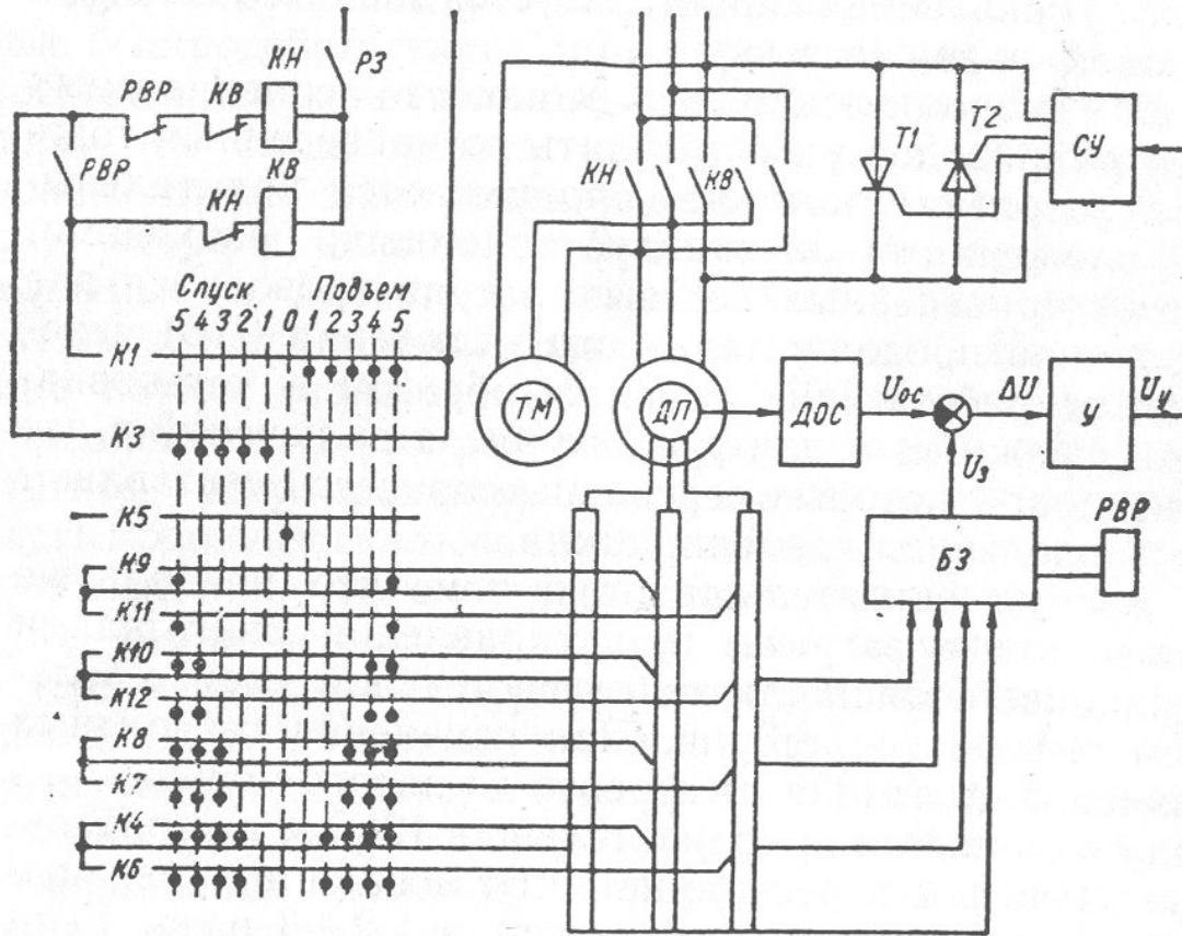
Схема тиристорного асинхронного электропривода, управляемого силовым контроллером ККТ-68А и соответствующие механические характеристики
