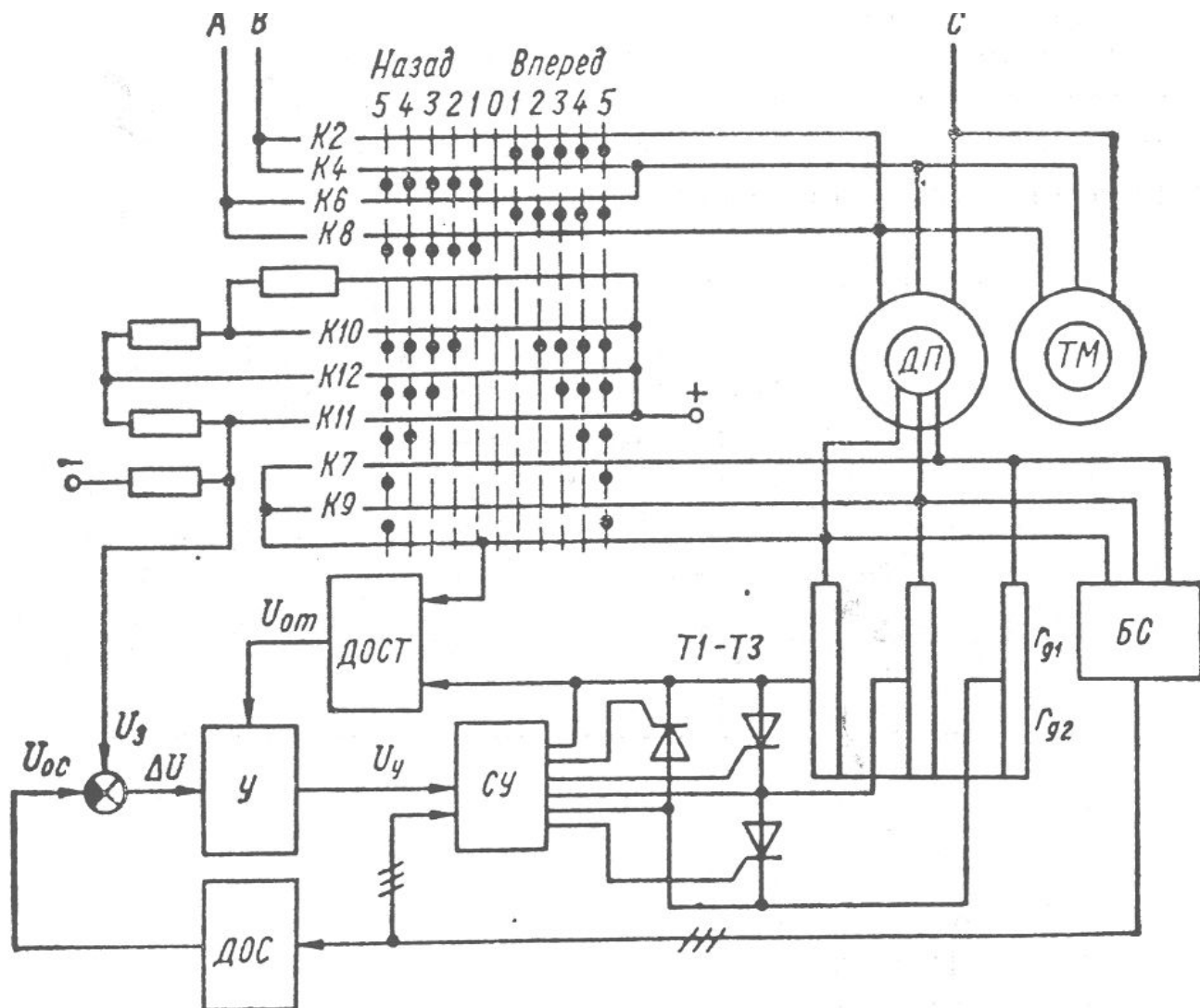
Схема контроллера ККР-61А, коммутирующего цепи статора и тиристорного регулятора тока ротора
