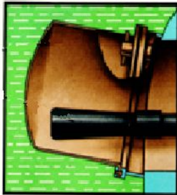
Уплотнение амбразуры спаренного пулемета
