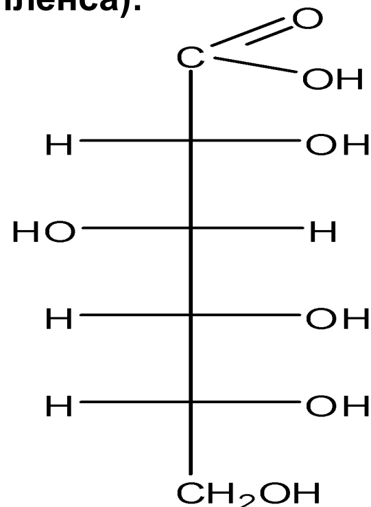
Глюконовая кислота
