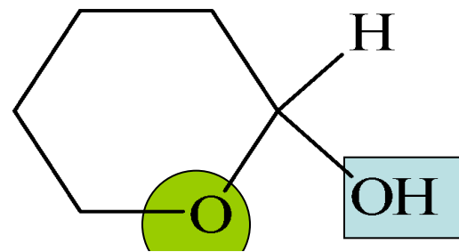
Полуацеталь
