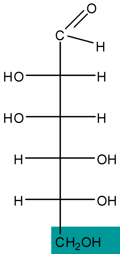
D-глюкоза
