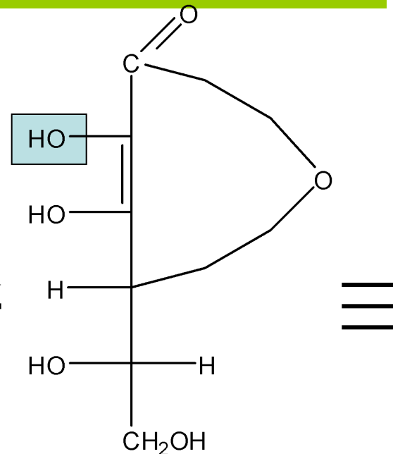
аскорбиновая кислота
