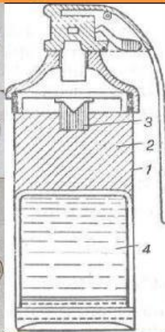
Современная американская ручная зажигательная граната: 1 - корпус; 2 - термит; 3 - термитный воспламенитель; 4 - коробка с отвержденным горючим
