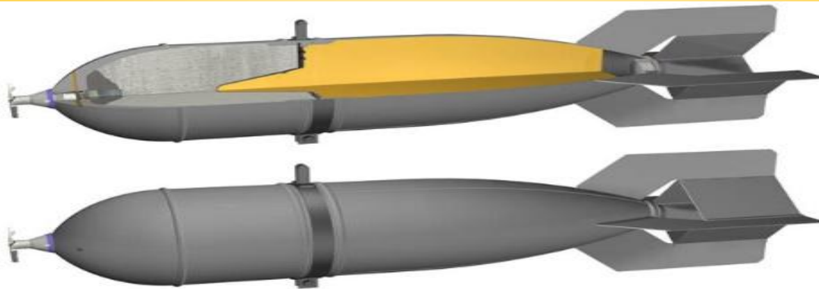
Зажигательная авиационная бомба с твердым горючим ЗАБ-50тг индекс 7-3-251 чертеж 3-0445 (1938г.)
