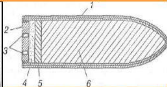
Электронно-термитная ружейная граната: 1 - корпус из электронного сплава; 2 - пробка из электронного сплава; 3 - газоотводящие отверстия (они же отверстия воспламенения); 4 - воспламенительный состав; 5 - переходный состав; 6 - термит
