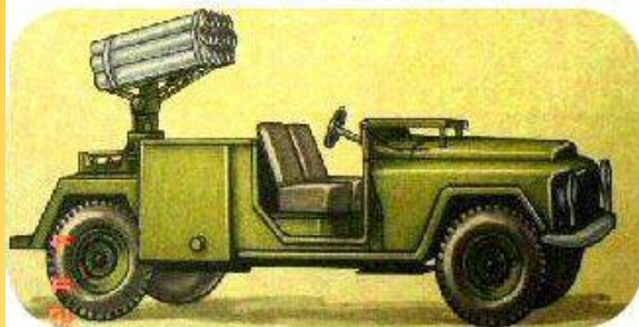
213мм зажигательный НУР
