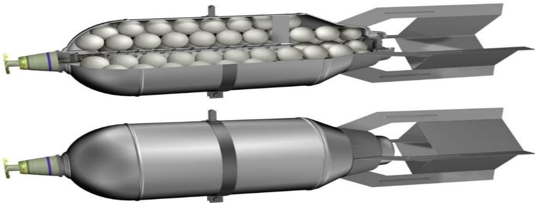
Зажигательная авиационная бомба с термитными шарами ЗАБ-100-65тш индекс 8-3-157 чертеж 3-01026 (1941г.)
