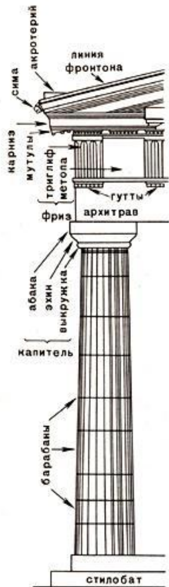
дорический ордер
