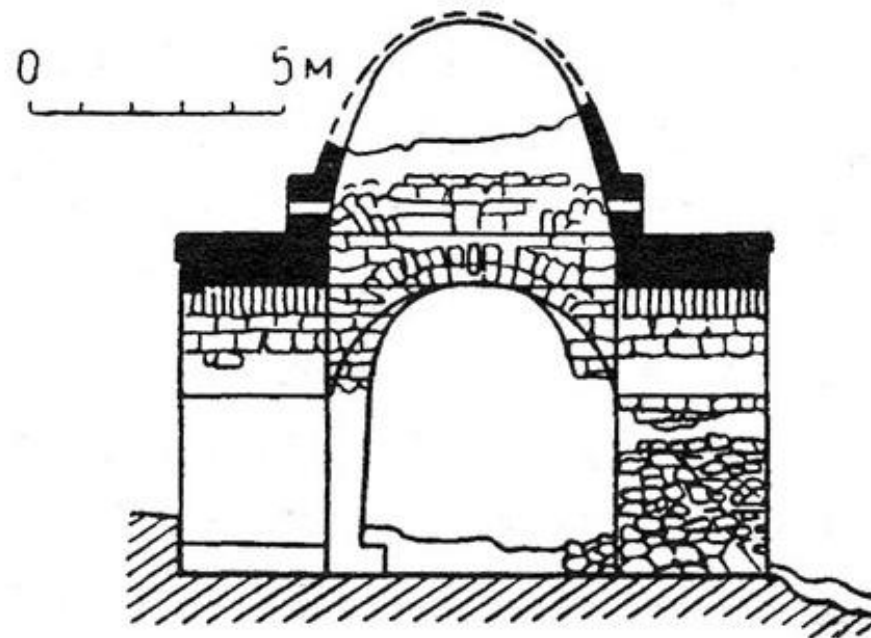
Чортак в Нейсаре. Внешний и внутренний вид, план, разрез
