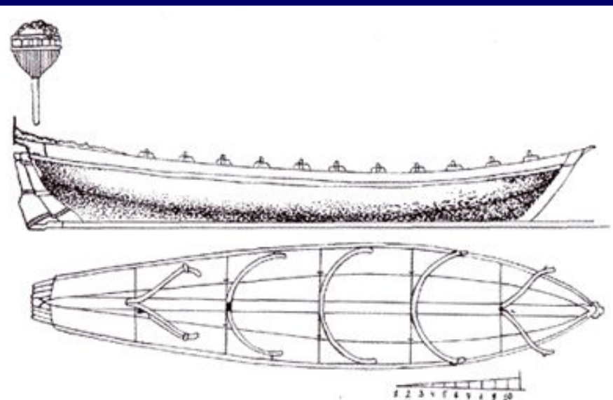
Рис. 6. Чертеж профилей ботика XVIII в.
