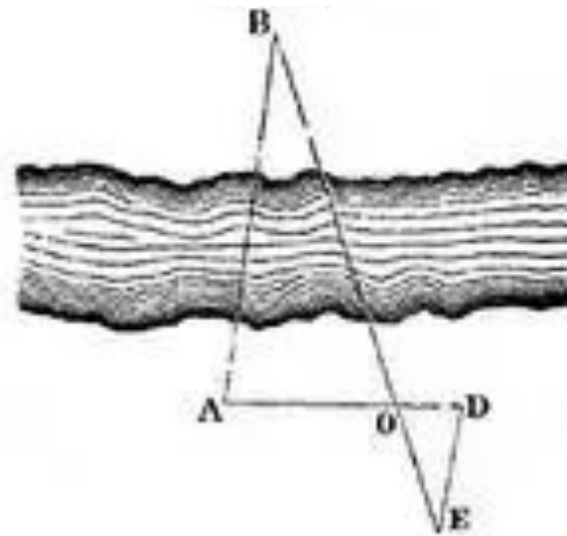
Измерение расстояния до труднодоступной точки
