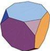
Усеченный куб
