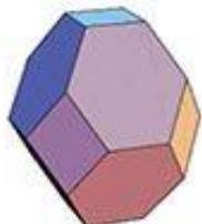
Усеченный октаэдр
