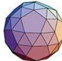
Курносый додекаэдр
