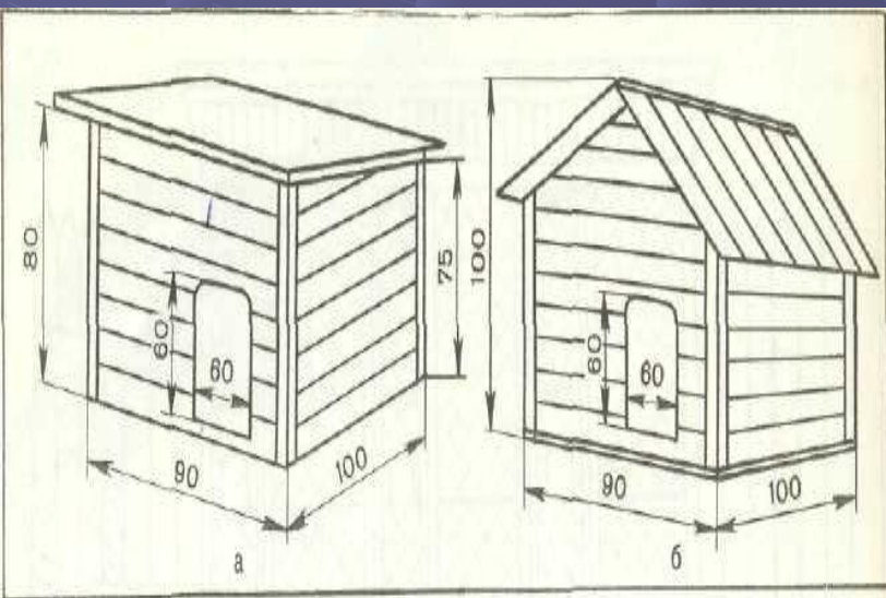
Будки для содержания собак: А-односкатная; Б- двухскатная (размеры даны в сантиметрах)
