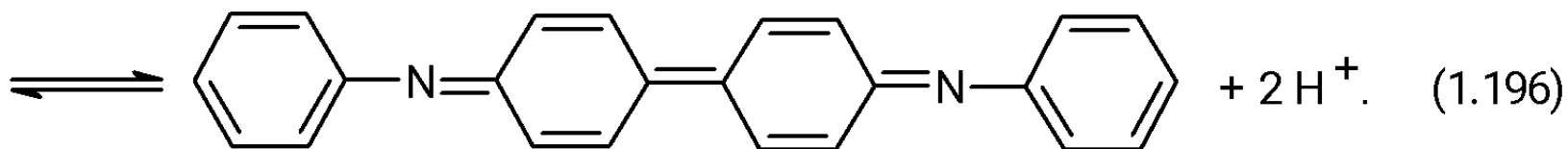
дифенилдифенохинондиимин (синий)
