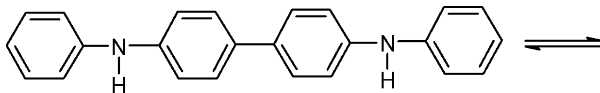
дифенилбензидин (бесцветный)
