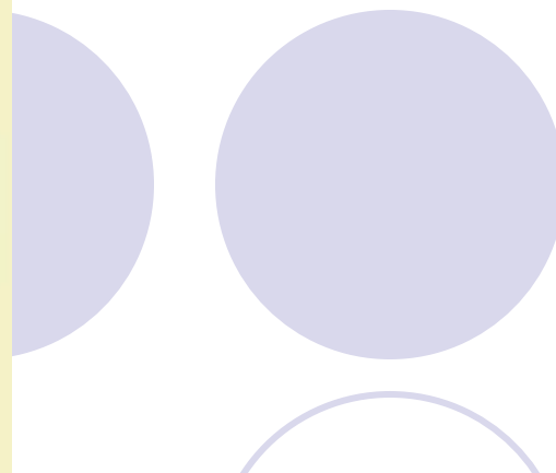
Уран
