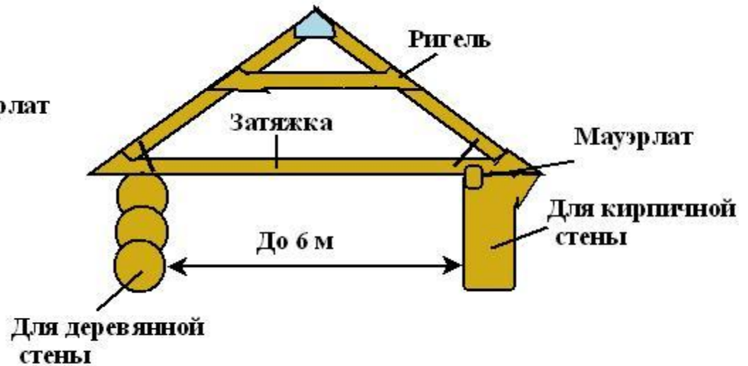
Простые висячие стропила с ригелем.
