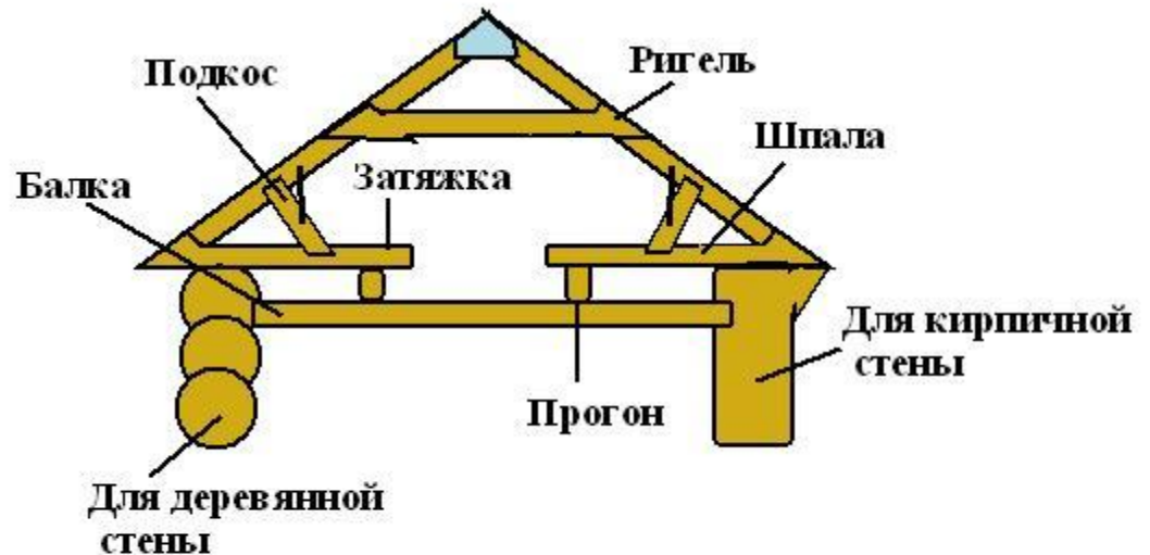
Висячие стропила со шпалами.
