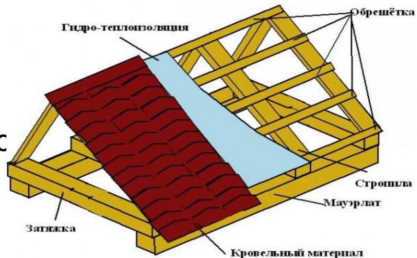
Конструкция двухскатной крыши.
