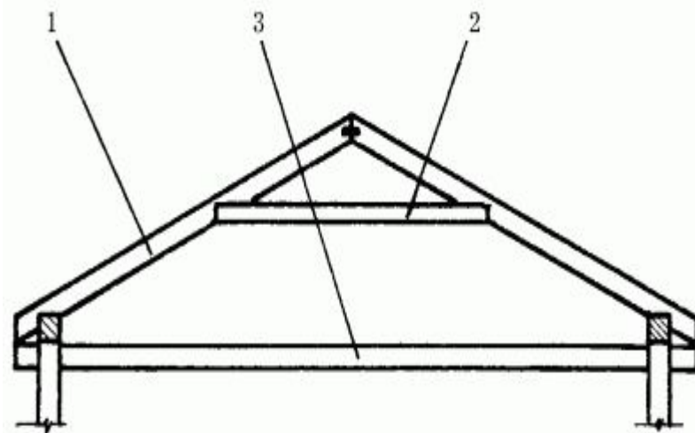
Наслонные стропила: (1) - стропильная нога; (2) - ригель; (3) - чердачное перекрытие
