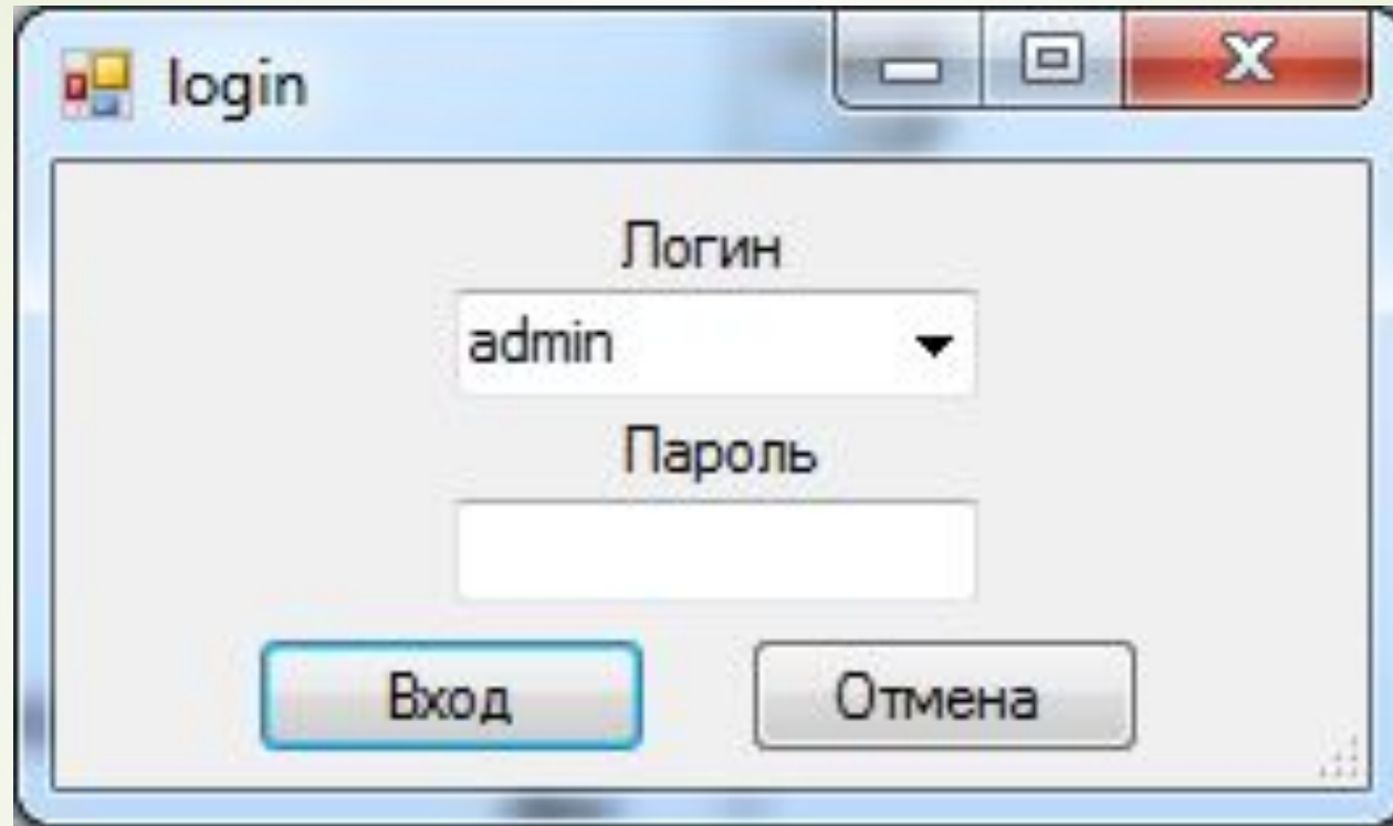
Окно авторизации
