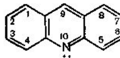
акридин
