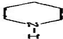
пиперидин
