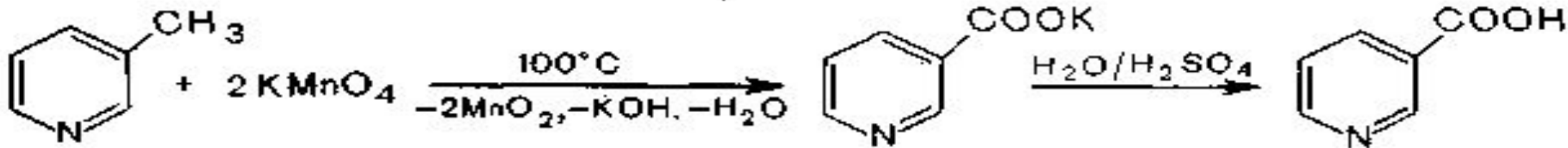
β-пиколин
