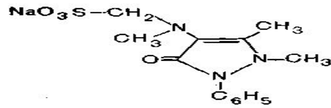
анальгин
