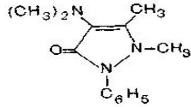
амидопирин
