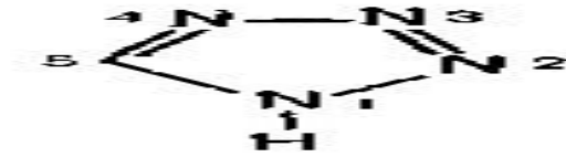
тетразол
