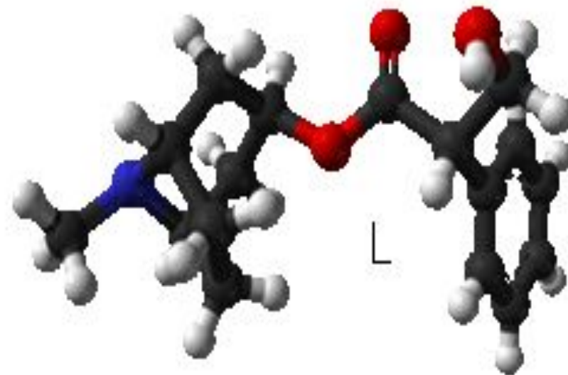
Атропин
