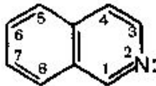
изохинолин
