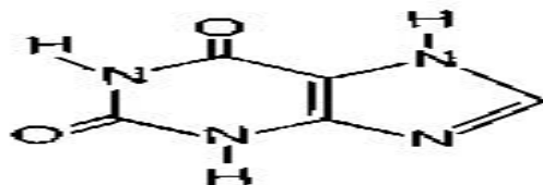
ксантин
