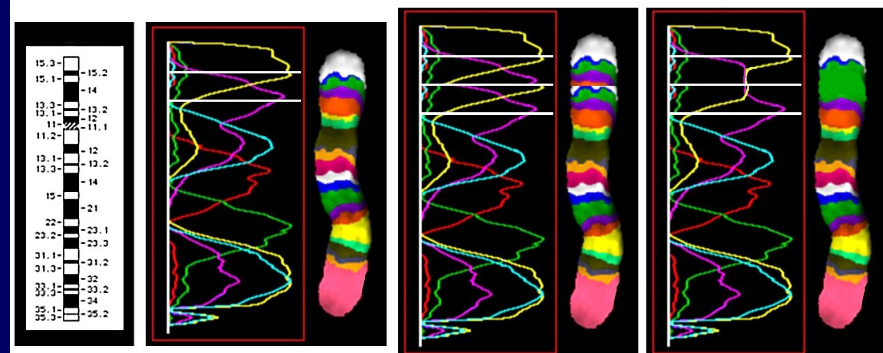
Дупликация 5p15.1-p14
