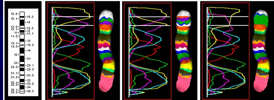
Дупликация 5p15.1-p14
