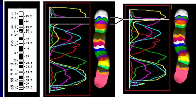
Инверсия 5p15.1-p14
