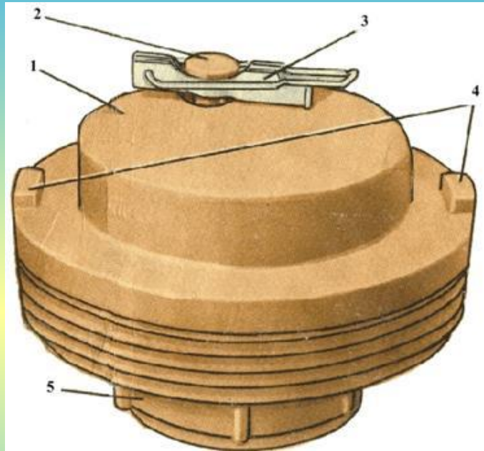
Взрыватель МВЧ-62
