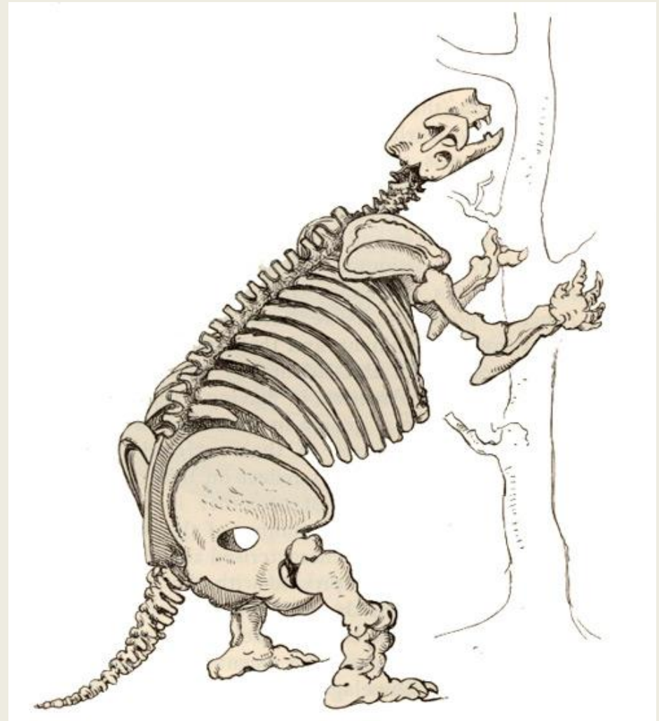
скелет милодона
