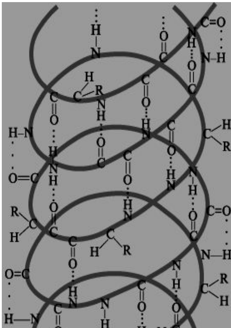
α-спираль
