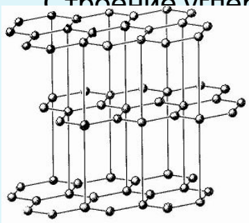
Строение углерода
