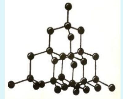
Строение кварца
