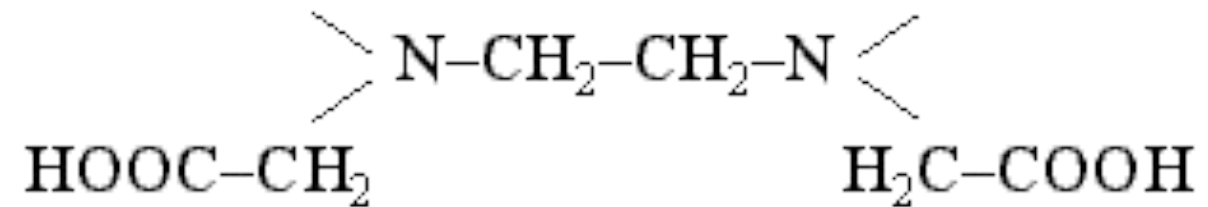
этилендиаминтетрауксусная кислота
