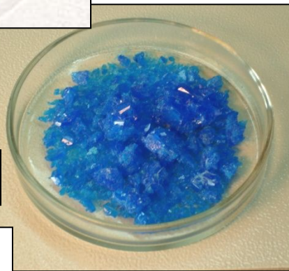
Медный купорос
