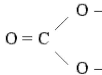
карбонат-ион
