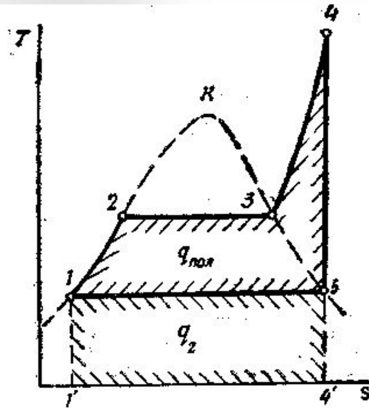
Рис. 10-25. Изображение теплофикационного цикла на диаграмме s-T
