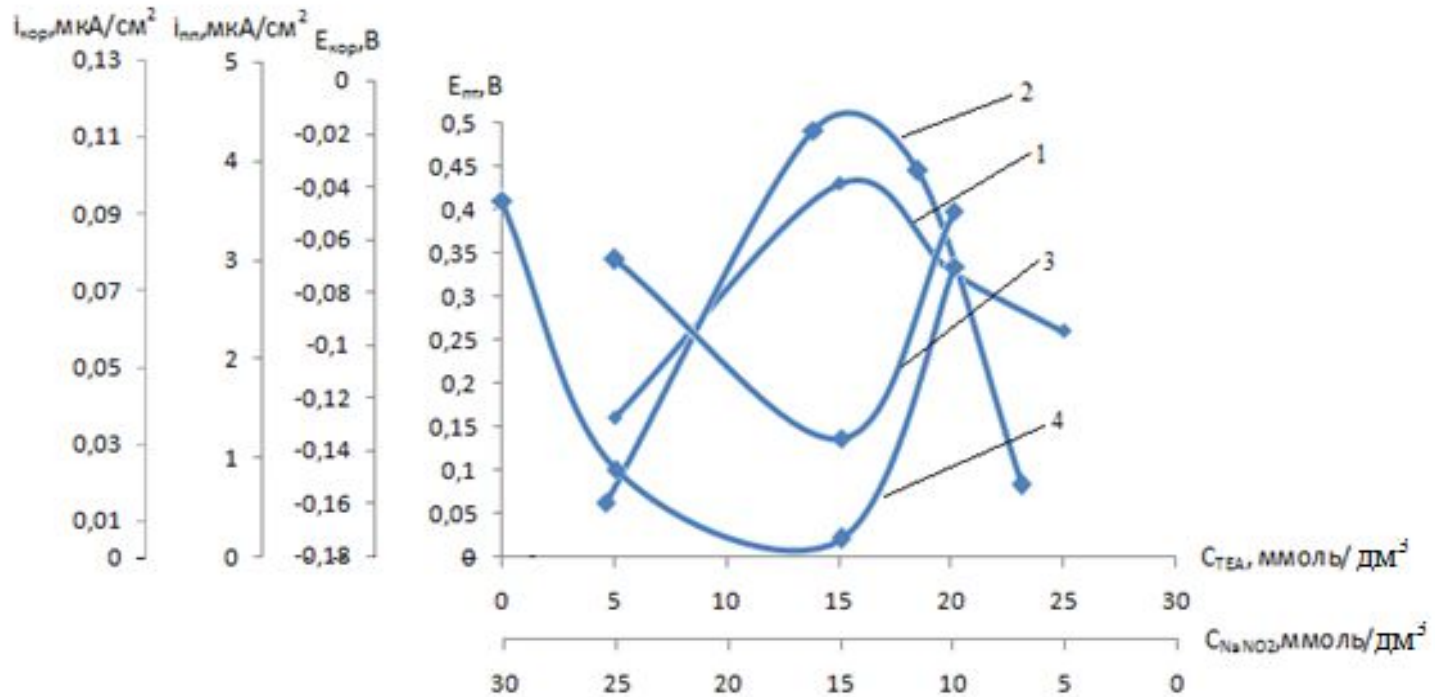
Рис. 5. Залежність електрохімічних параметрів анодної поведінки сталі у водно-сольовому розчині від співвідношення концентрації компонентів у сумішах ТЕА- NaNO_2 зі сталюю сумарною концентрацією 30 ммоль/дм 3 (ізомольярні серії): 1 – потенціал пітінгоутворення ( E_{пт} ); 2 – корозійний потенціал ( E_{кор} ); 3 – густина струму повної пасивації ( i_{пп} ); 4 – струмовий показник швидкості корозії ( i_{кор} , обчислений на підставі масометричних вимірювань )
