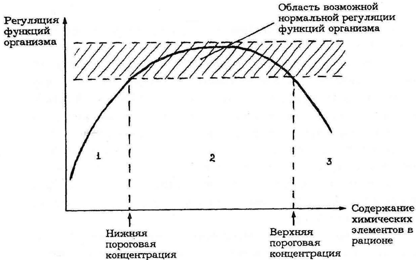
Рис. 7. Зависимость регуляторных процессов в организме от содержания химических элементов в рационе (по В.В. Ковальскому, 1976)
