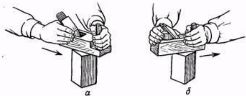
Рис. 22. Строгание торца от себя ( a ) и на себя ( б )
