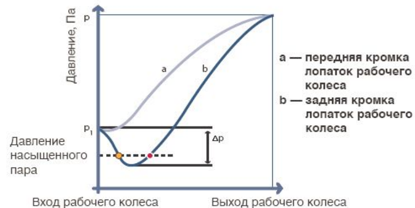
Рис. 2.2.10: Изменение давления в центробежном насосе
