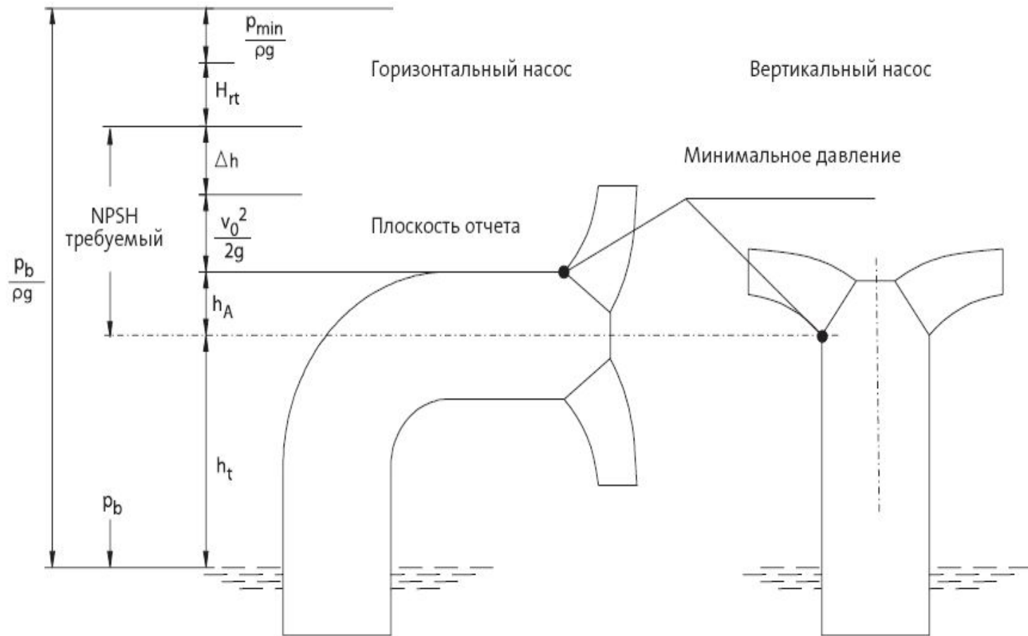
Рис. 9 Размеры и давления для расчета NPSH
