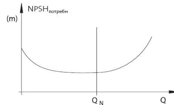
Рис. 11 Типичное распределение требуемого значения параметра NPSH по отношению к расходу потока в насосе.
