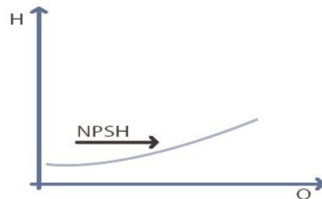
Рис. 2.2.12: NPSH характеристика
