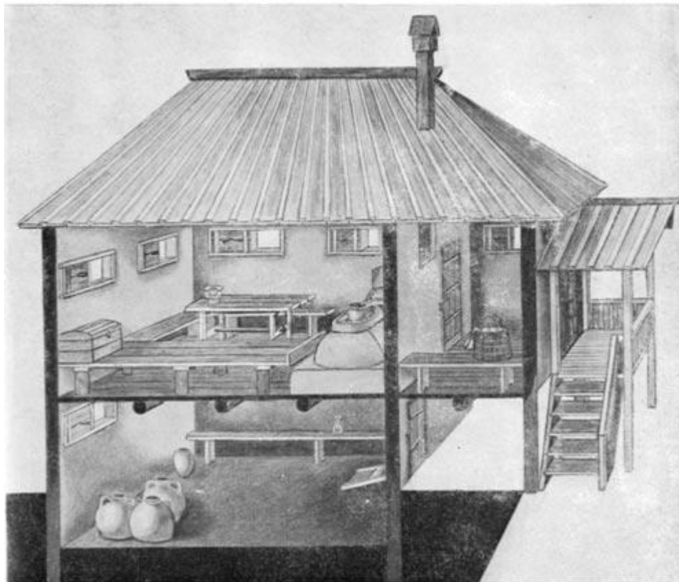
Давньоруський будинок каркасно-стовпової конструкції (реконструкція)
