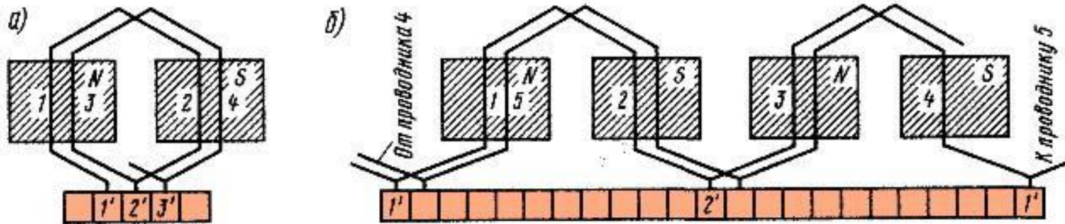
Рис. 16. Петлевая (а) и волновая (б) обмотки якоря
