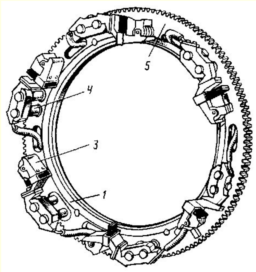
Рис. 19. Щеткодержатель тягового двигателя
