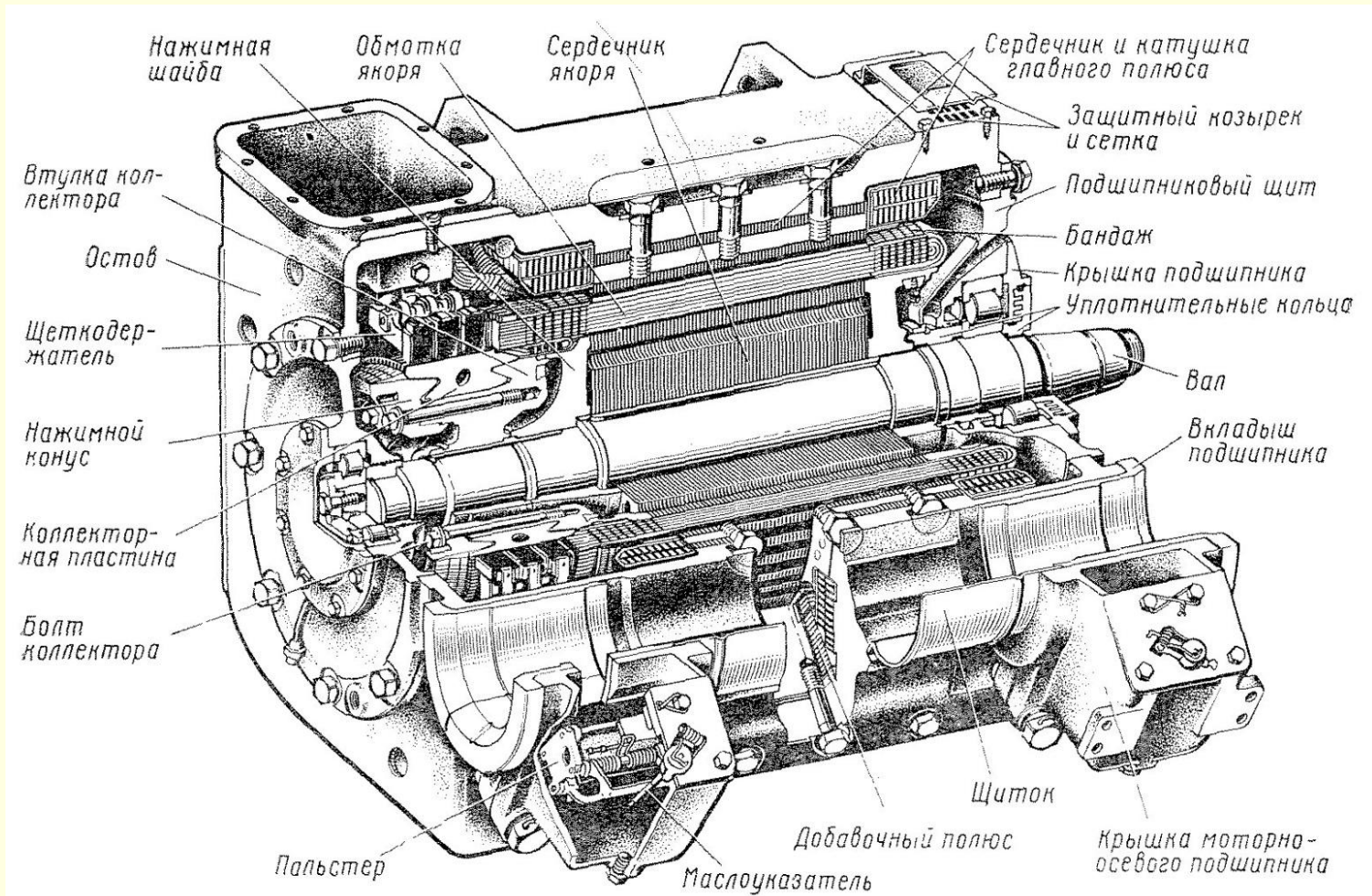
Тяговый электродвигатель тепловоза 2ТЭ10Л
