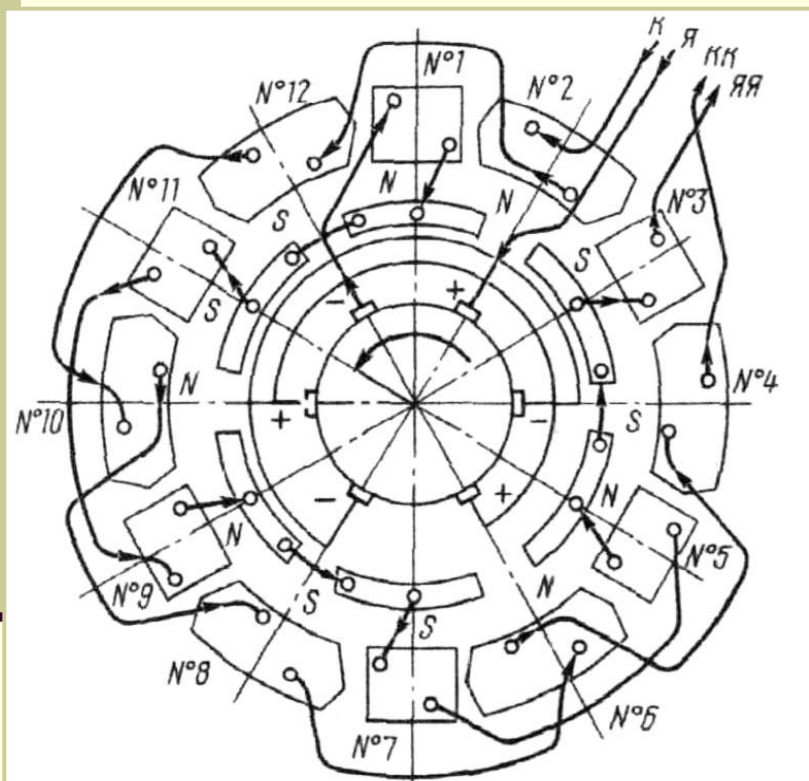
Схема соединения обмоток тягового двигателя НБ-418К6
