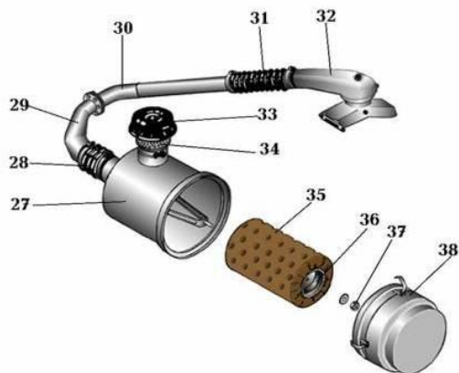
СИСТЕМА ПИТАНИЯ ДВИГАТЕЛЯ ВОЗДУХОМ
