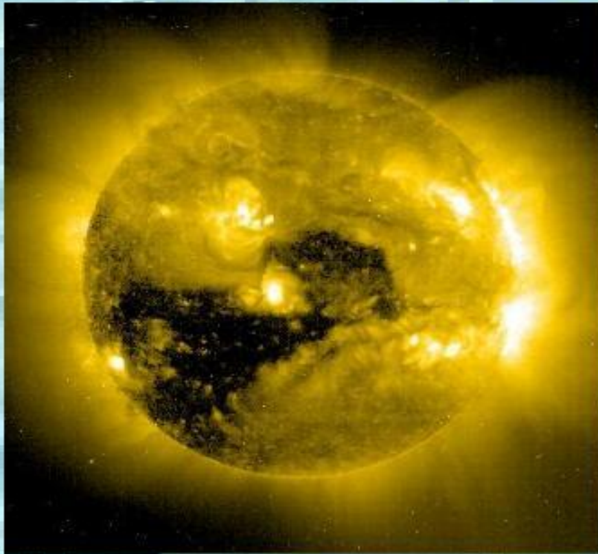
Фотография Солнца в диапазоне мягкого рентгеновского излучения. Корональные дыры проявляются в виде тёмных образований.
