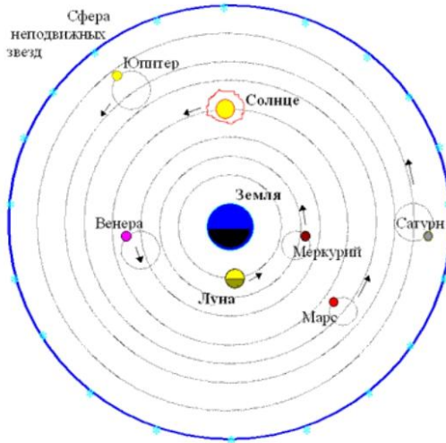
Геоцентрическая система мира
