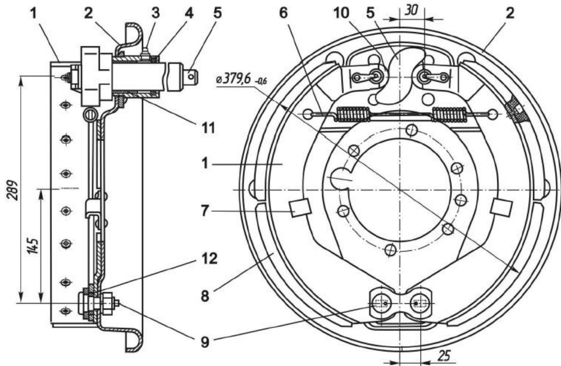
Тормозной механизм автобуса ПАЗ-32053-04
