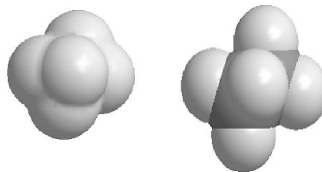
Модель молекулы бутана (а) и поверхность доступная растворителю с разрешением 40 (б)
