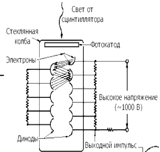
Рис. 2. Устройство ФЭУ
