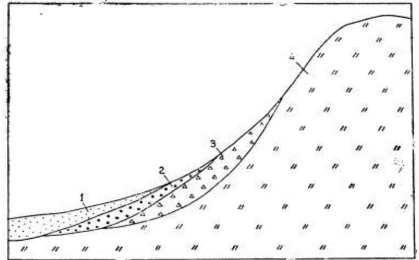
Рис. 3. Делювиальные отложения на склоне холма: 1 — тонкие; 2 — средние; 3 — грубые, 4 — Коренная порода
