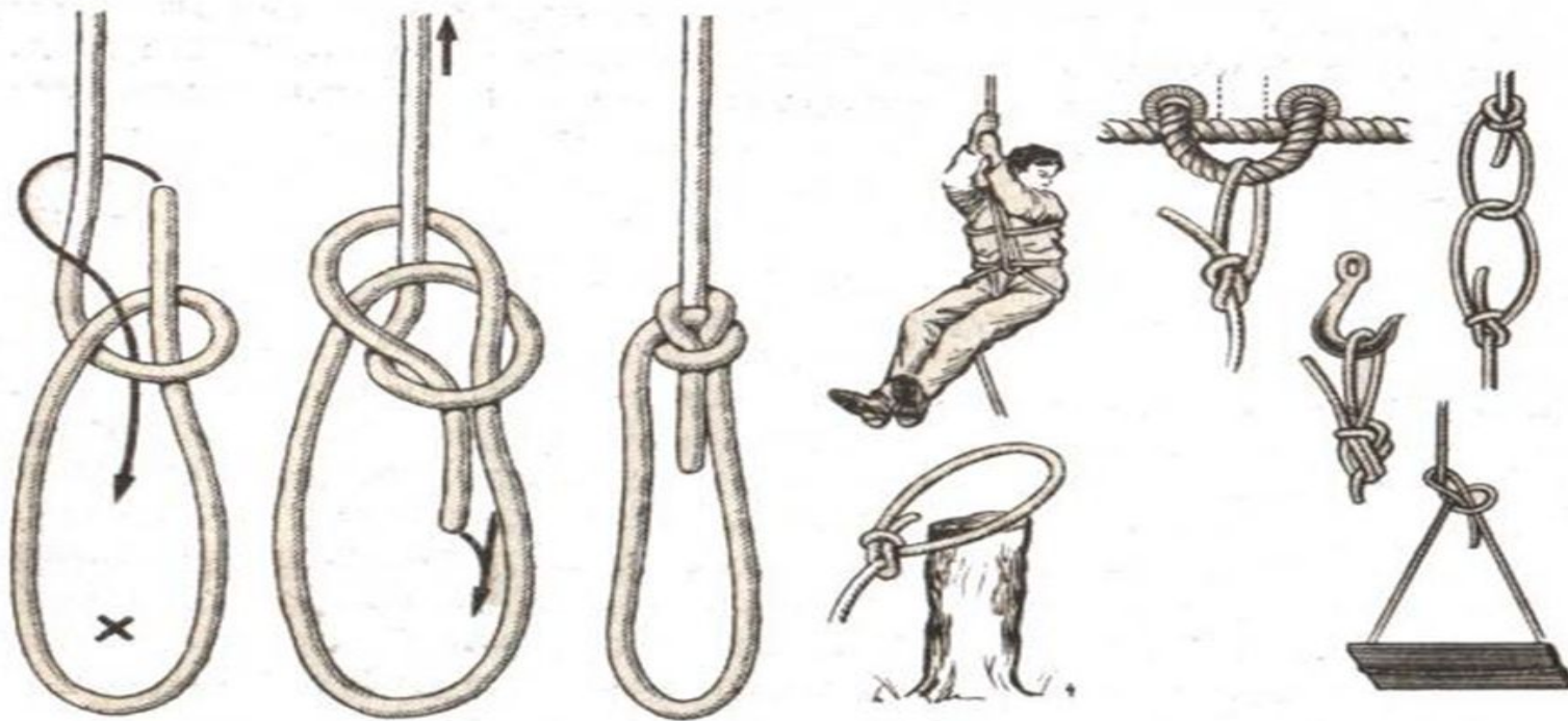
Беседочный узел
